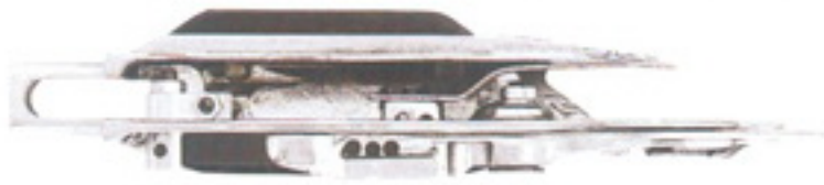
多尼尔 I-II 送剑 Sending Gripper-Dornier I-II
